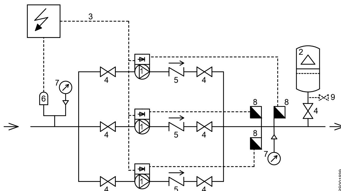
Figure 7: Système à pompes multiples
