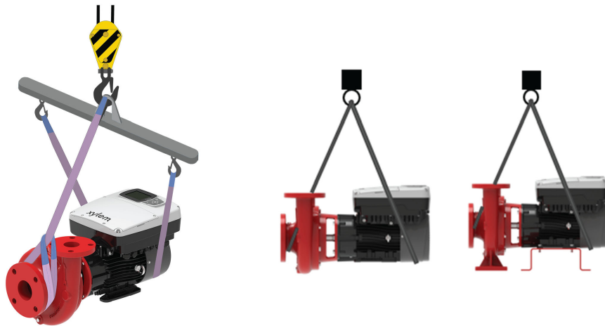
Méthodes de levage acceptables pour les modèles à aspiration directe e-1531X et e-1532X
