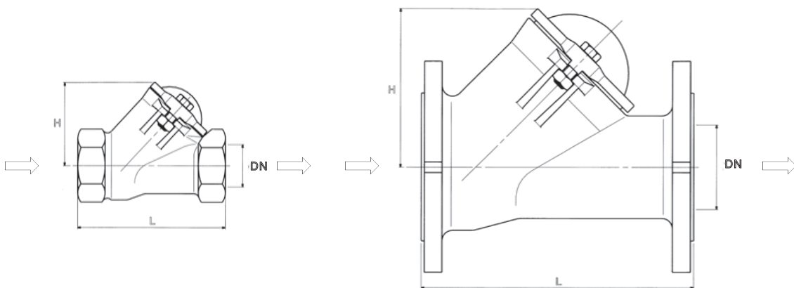
MODELL Rp 1 1/4 - 1 1/2 - 2
