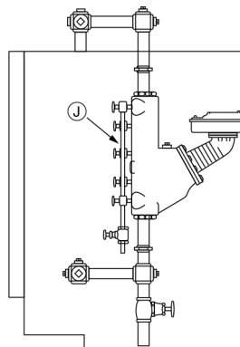
Figura 41: Todos los otros modelos
