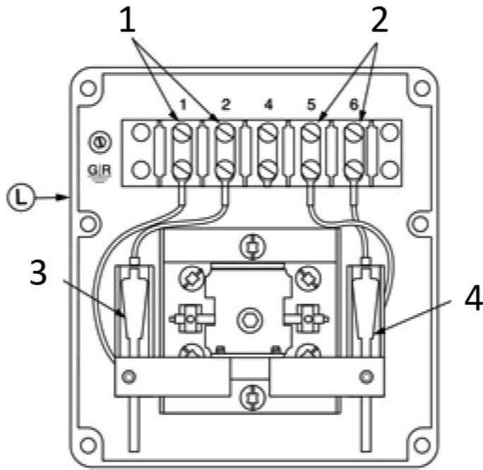
Figure 32: Modèle à réinitialisation automatique 159S
