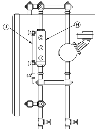
Figure 24: Tous les autres modèles
