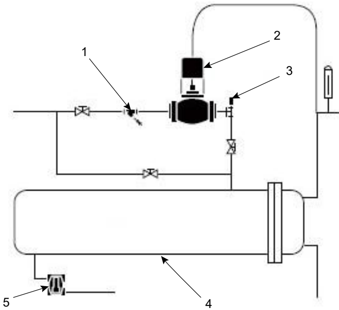
Figura 3: Calentador de agua sin tanque
