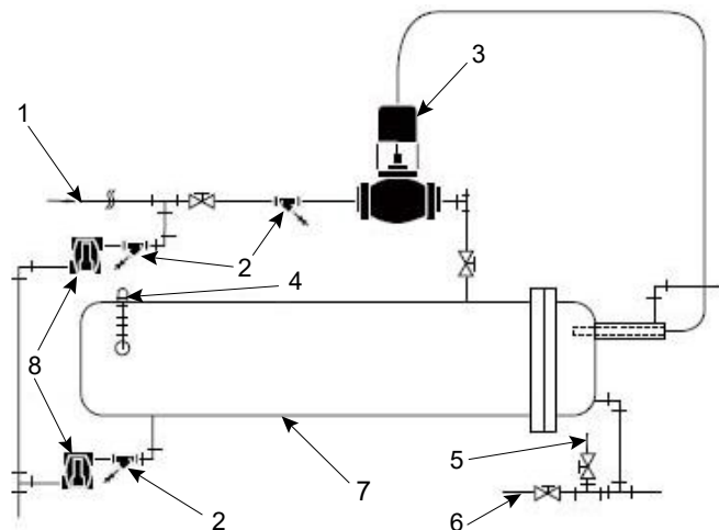
Figure 1: Chauffe-eau à la vapeur
