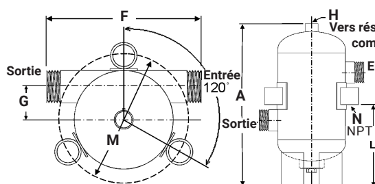
Modèles 3 po (76,2 mm) avec crépine et supports en option
