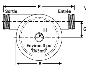
Modèles 3 po (76,2 mm) avec crépine
