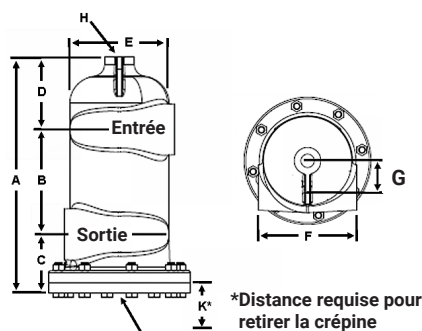
Modèles 2 po et 2 1/2 po (50,8 mm et 63,5 mm) avec crépine
