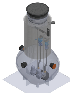
C-XL5P-DC-XXX-35/X Pumpbrunn Flygt Compit XL5-35. Höjd 3500mm för dn 50 pumpar. Vikt exkl. pumpar: Ca 360 Kg. Yttre Volym ca: 4000L Produktkod: 01-45 90 27
